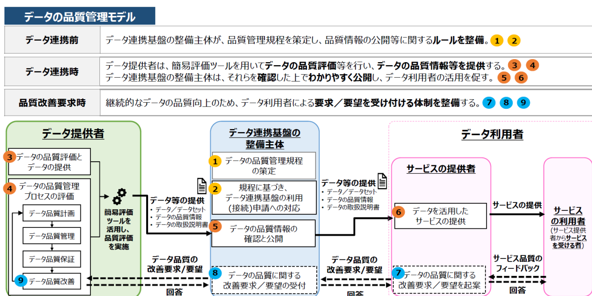
図 5-4 データの品質管理モデル
